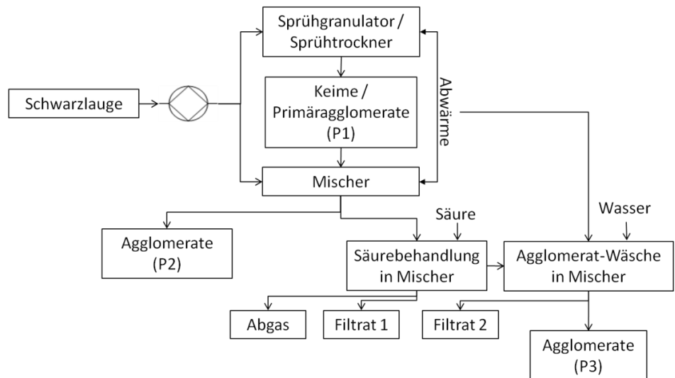
Abb.: Herstellung von Lignin-Agglomeraten aus der Ablauge eines Zellulosegewinnungsprozesses
