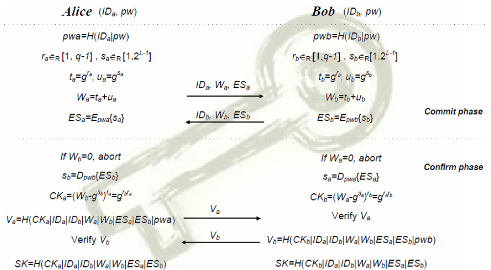
Abb.: Ablauf des Verschlüsselungsverfahrens
